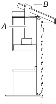
A. Conduit circulaire de 10 po (25,4 cm) B. Bouche de décharge sur toit
