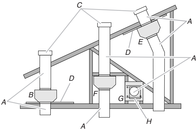
A. Conduit circulaire de 10 po (25,4 cm) B. Montage au-dessus des solives C. Bouches de décharge sur toit D. Contreplaqué (facultatif pour certaines installations) E. Montage sous les chevrons F. Montage sur traverses de ferme G. Conduit horizontal, montage sur traverses de ferme H. Bouche de décharge murale
