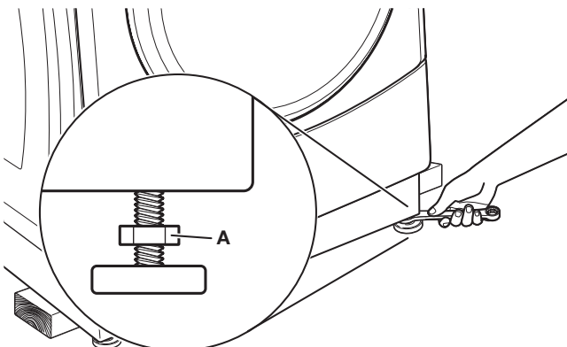
A. Contre-écrou
