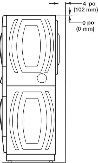
Distances de dégagement arrière/sur le dessus
