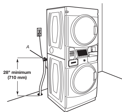
A. Brise-siphon
