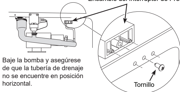
Ensamble del Interruptor de Presión
