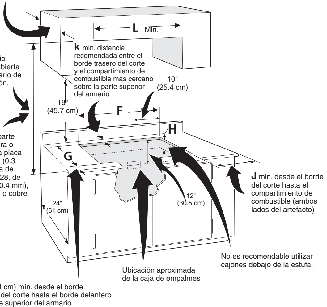
Figura 2 – EL CORTE DE LA PARTE SUPERIOR DEL ARMARIO
