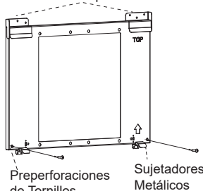
Figura C (El motor simple se verá diferente) Soportes Metálicos
