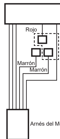
Configuración del Cableado Aumentado Máx. de 390 CFM
