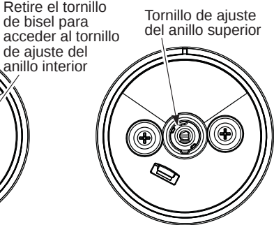
Tornillo de ajuste del anillo superior del quemador apilado de llama doble para llama únicamente (sin ajuste del anillo inferior)
