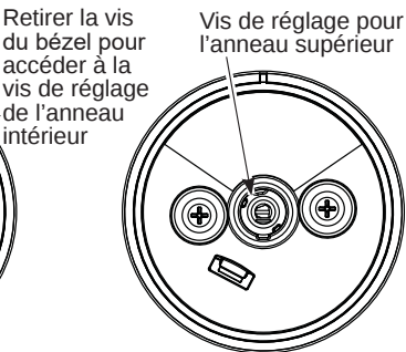
Retirer la vis du biseau pour accéder à la vis de réglage de l'anneau intérieur Vis de réglage pour l'anneau supérieur
