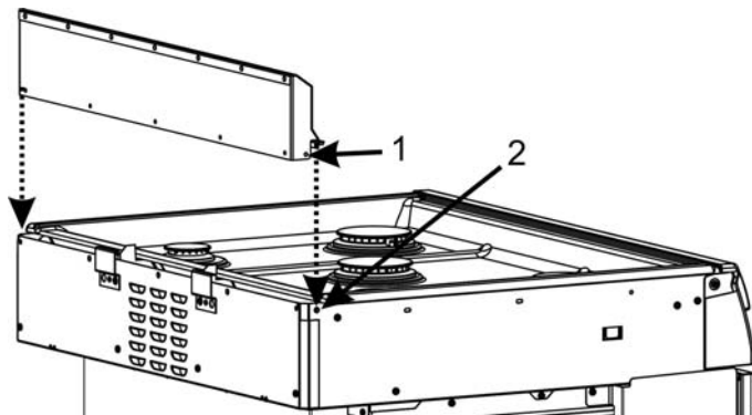
Figure 7 : Positionnement du dossier bas
